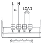
Рис. 6 - Подключение датчика MS-24B
