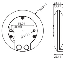
Рис. 1 - Габаритные и установочные размеры MS-24B
