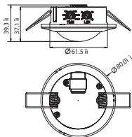
Рис. 2 - Габаритные и установочные размеры MS-25B встраиваемого исполнения
