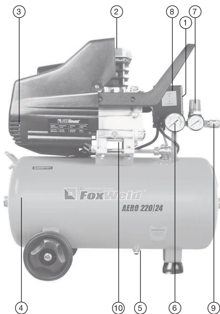
AERO 220/24 AERO 220/50
