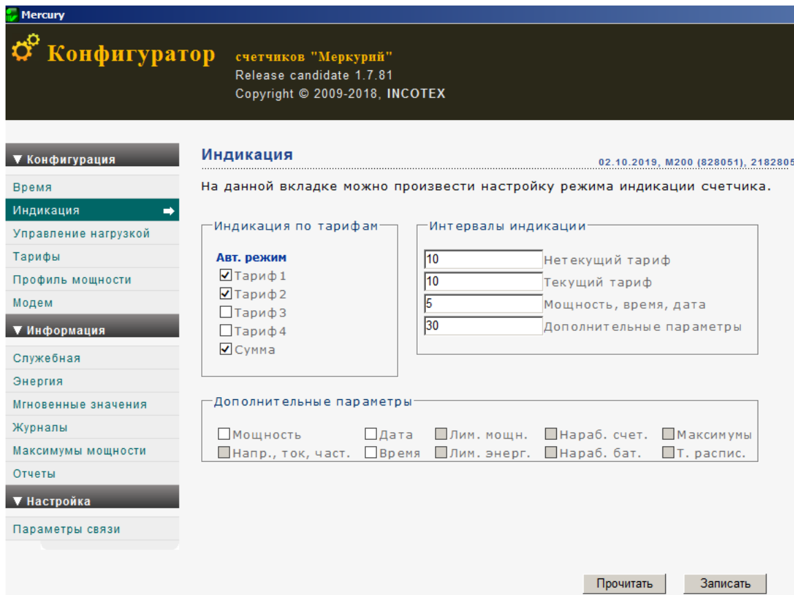
Рисунок 4.4 – Вкладка «Индикация»
