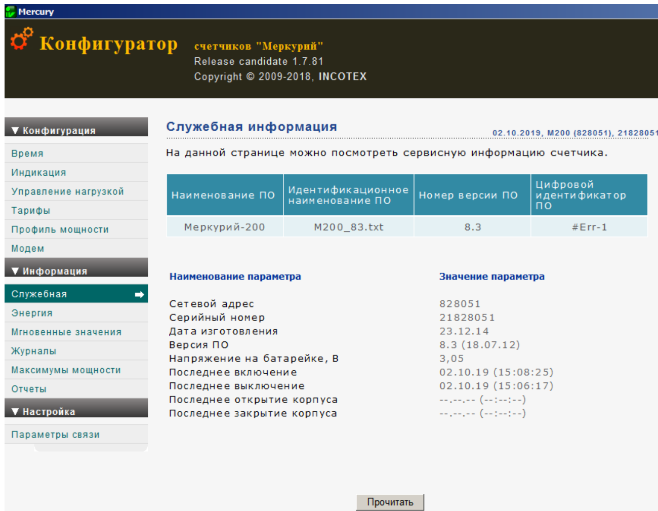
Рисунок 4.2 – Вкладка «Служебная»
