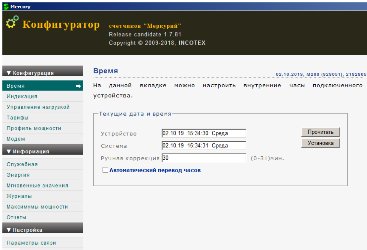
Рисунок 4.3 – Вкладка «Время»
