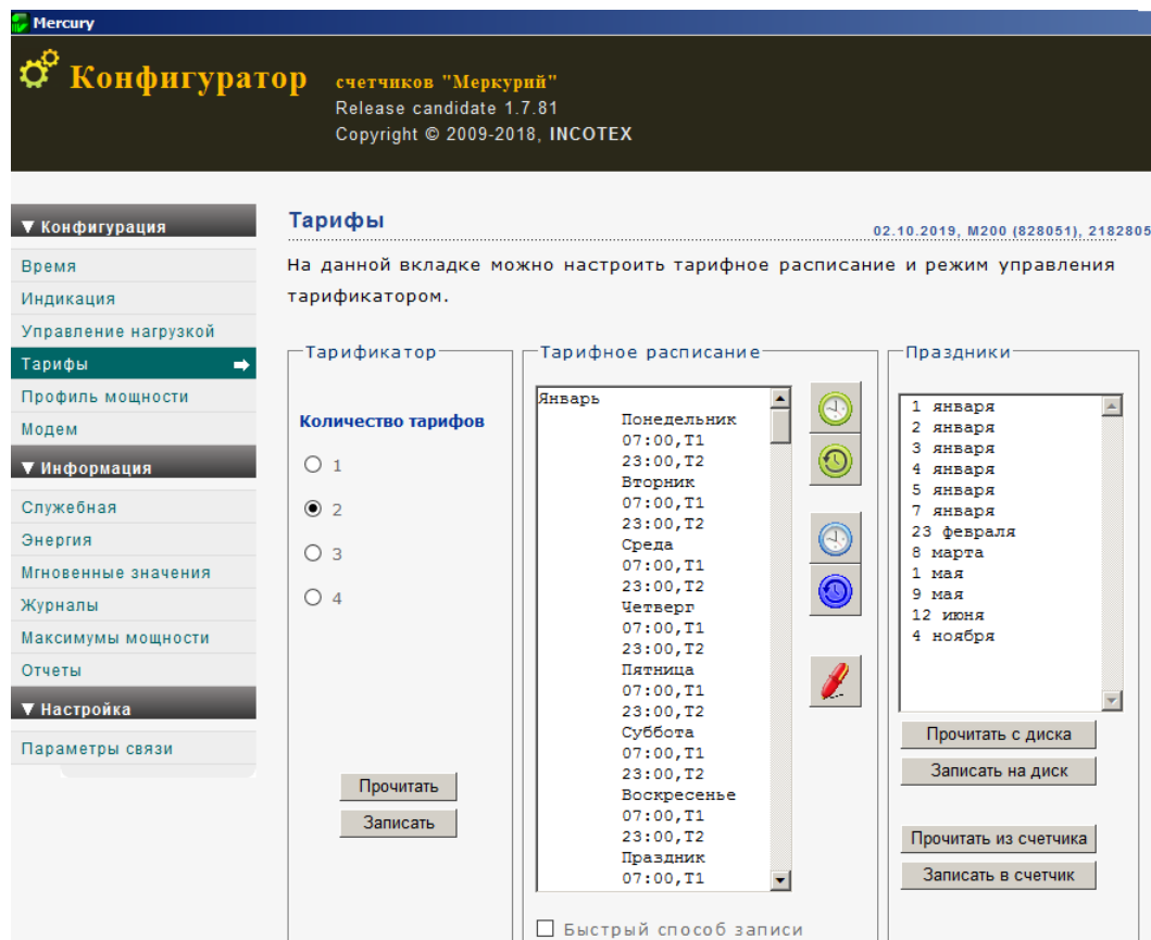
Рисунок 4.5 – Вкладка «Тарифы»
