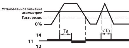
Рисунок 7. Схема работы реле РН (кроме моделей РН-04, РН-05) при асимметрии фаз
