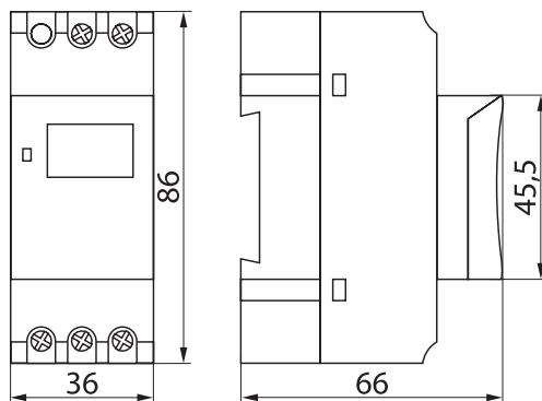
Рисунок 2. Габаритные и установочные размеры таймера ТЭ-АС, мм
