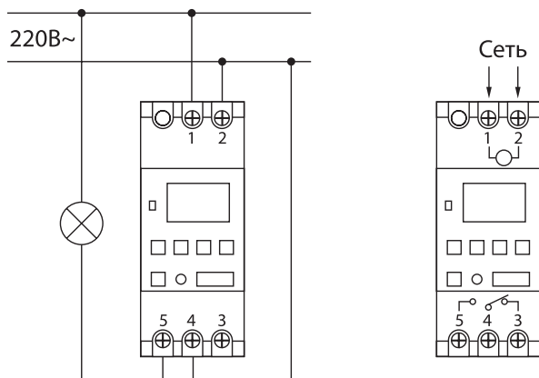
Рисунок 3. Электрическая схема подключения таймера ТЭ-АС
